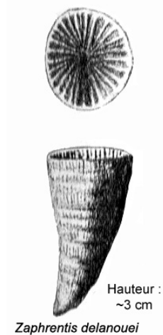
FIG. 5 – Zaphrentis delanouei , Rugueux solitaire du Carbonifère.
