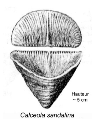
FIG. 3 – Calceola sandalina , Rugueux solitaire Dévonien de forme caractéristique, qui présente la particularité d'avoir un opercule.
