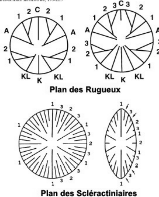
FIG. 6 – Développement comparé des septes chez les Rugueux et les Scléractiniaires.
