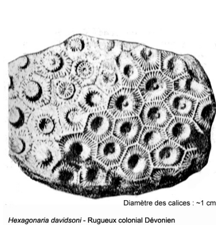
FIG. 4 – Hexagonaria davidsoni , Rugueux colonial Dévonien.
