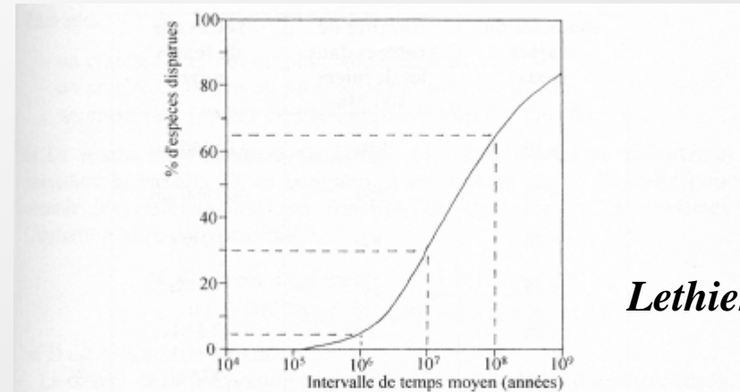
FIGURE 58 : Courbe des exterminations pour le Phanérozoïque, donnant le % d'espèces disparues au cours d'une extinction en fonction de l'intervalle de temps séparant deux extinctions successives d'intensité égale ou supérieure (voir le texte). Par simplification, les marges d'erreurs de la courbe ne sont pas figurées (d'après Raup, 1992).
