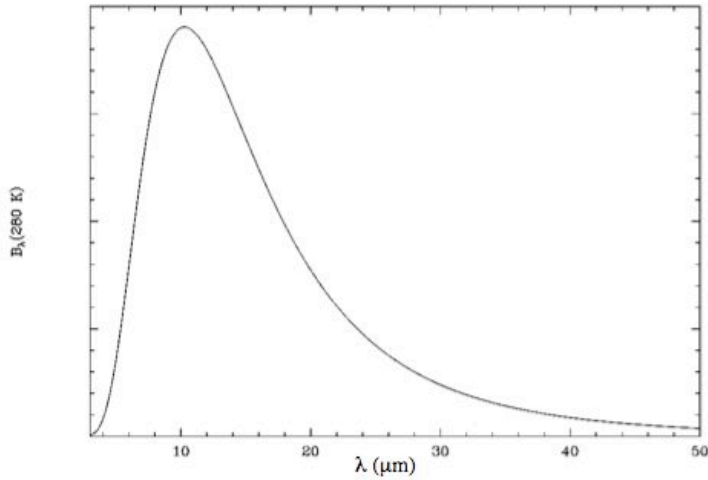
Rayonnement de corps noir à la température de la Terre
