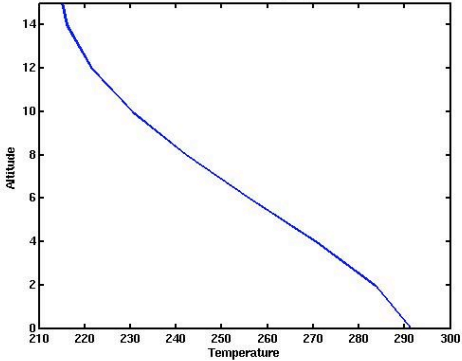
Temperature dans la troposphere
