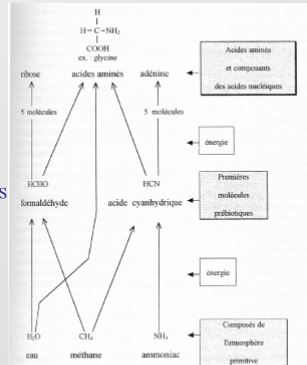
FIGURE 54 : Schéma des réactions possibles aboutissant aux premiers composés organiques importants.
