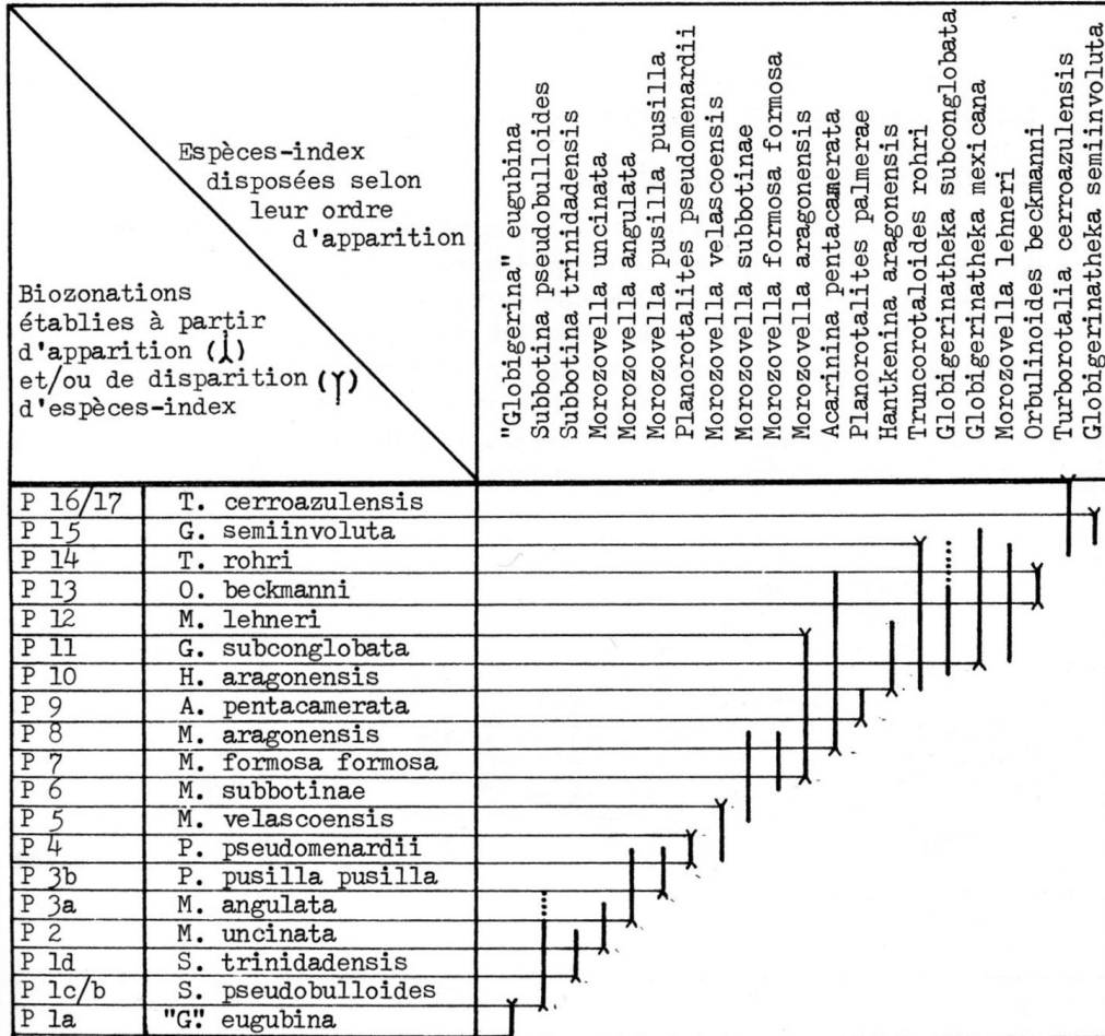
Figure 14.2 – Succession de quelques Foraminifères planctoniques du Paléocène et de l'Eocène, rangés par ordre d'apparition.
